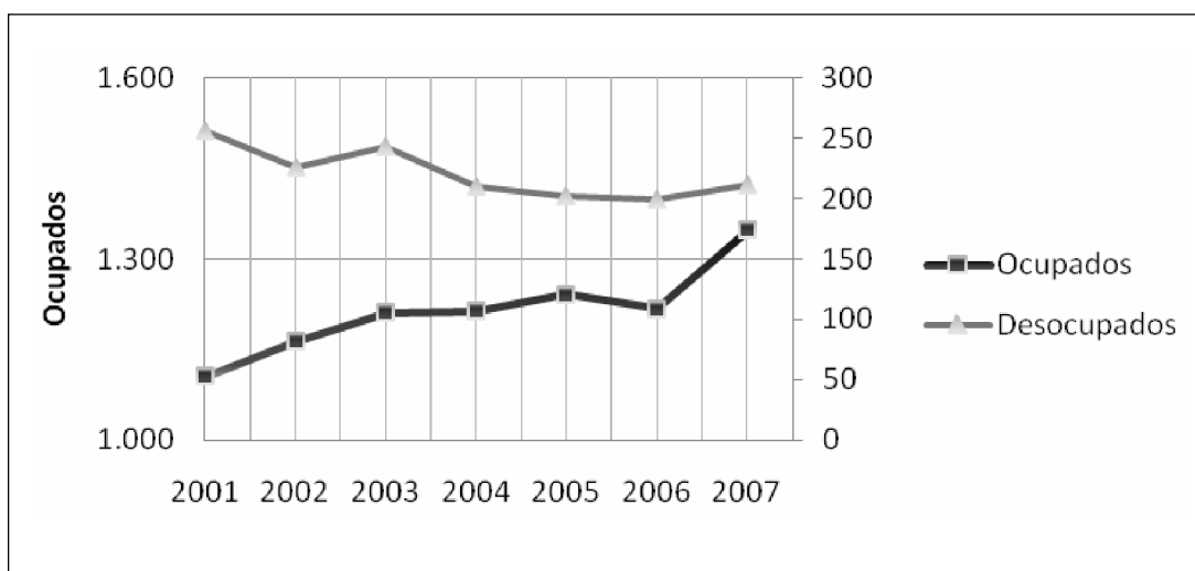
Gráfico 8. Ocupados vs. Desocupados en Medellín, 2000-2007.
